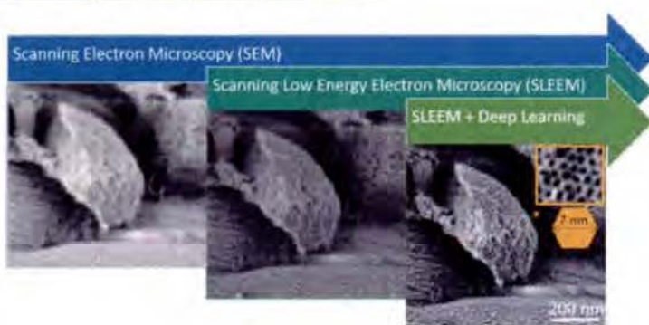
Obr. 12: Získávání strukturních informací o nanomateriálech pomocí pokročilé skenovací mikroskopie nízkonoenergetických elektronů ve spojení s hlubokým učením. Snímky SLEEM podpořené hlubokým učením ukazují vybrané detaily před a po „denoisingu“ demonstrováném na mezoporézním oxidu křemičitém.
