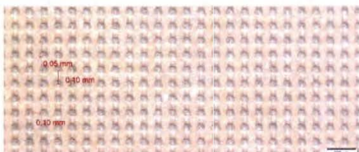
Obr. 14: Mikrostrukturovaný povrch korozivzdorné (austenitické) oceli.
